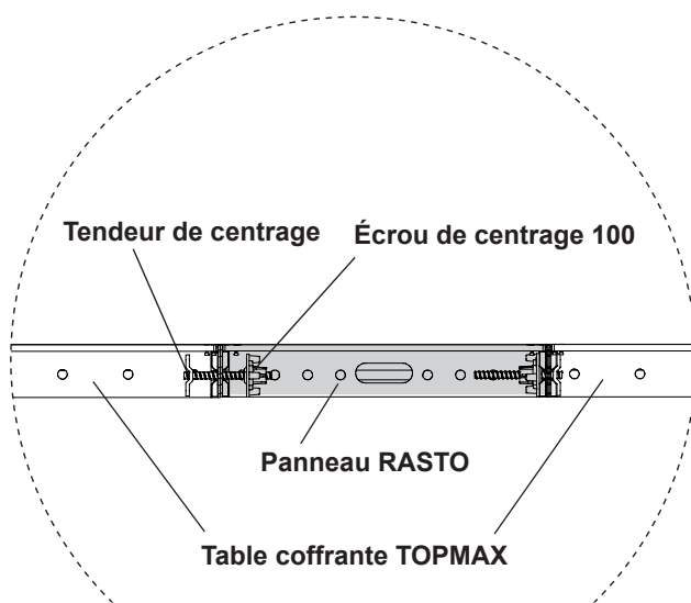
Vue latérale
