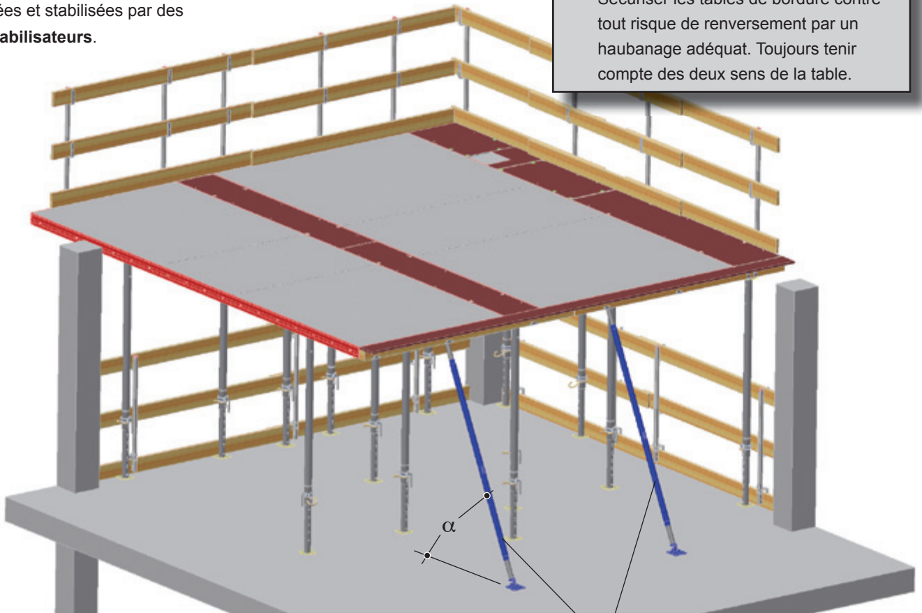
Étai stabilisateur
