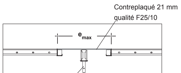
Bande d'ajustement à l'intérieur de la surface de plafond TOPMAX avec étaieiment central en cas d'utilisation d'une table de format 180 x 540
