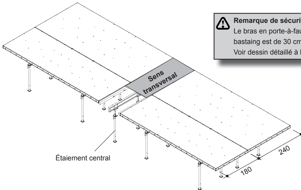
Bande d'ajustement à l'intérieur de la surface de plafond TOPMAX avec étaieiment central en cas d'utilisation d'une table de format 240 x 540
