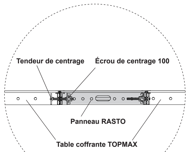
Vue latérale
