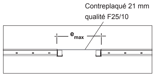
Bande d'ajustement à l'intérieur de la surface de plafond TOPMAX sans étaieement central en cas d'utilisation d'une table de format 240 x 540
