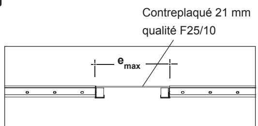
Bande d'ajustement à l'intérieur de la surface de plafond TOPMAX sans étaieement central en cas d'utilisation d'une table de format 180 x 540
