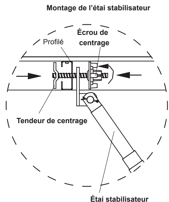
Étai stabilisateur
