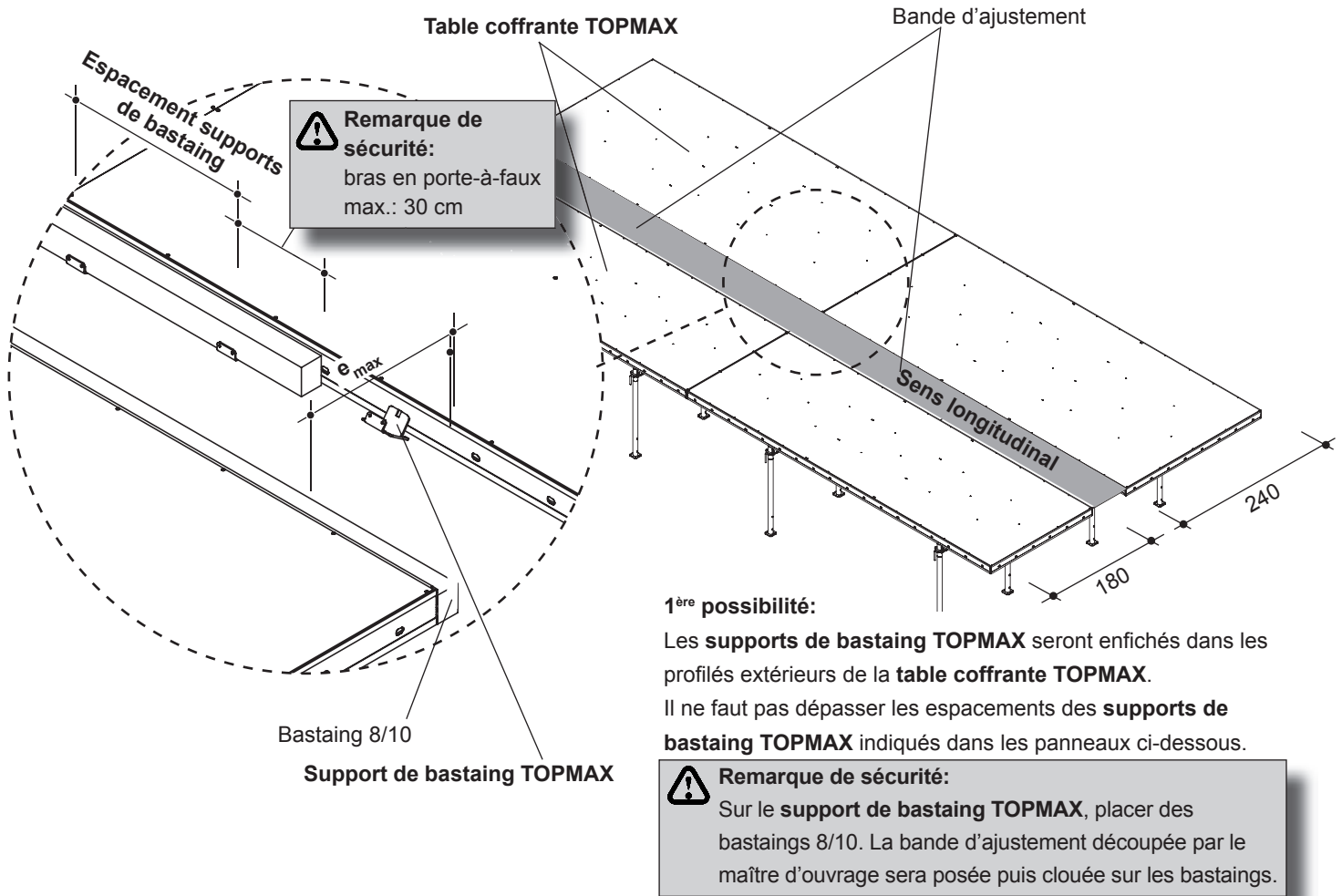
Bande d'ajustement à l'intérieur de la surface de plafond TOPMAX sans étaieement central en cas d'utilisation d'une table de format 240 x 540
