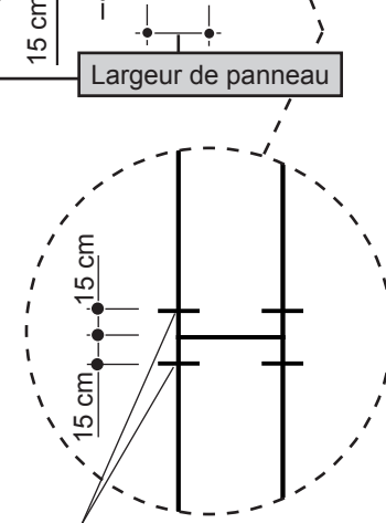
Tendeur de centrage + écrou de centrage
