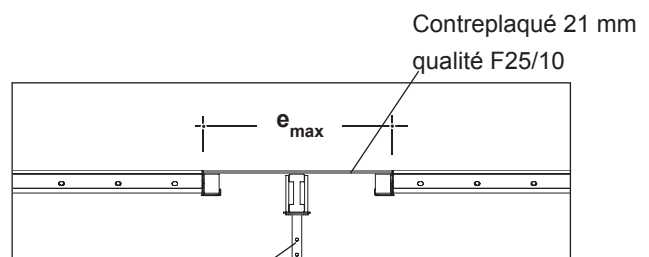
Bande d'ajustement à l'intérieur de la surface de plafond TOPMAX avec étaieiment central en cas d'utilisation d'une table de format 240 x 540
