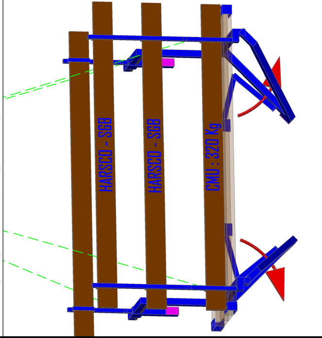
4. Elingage et dépliage des jambes de force
