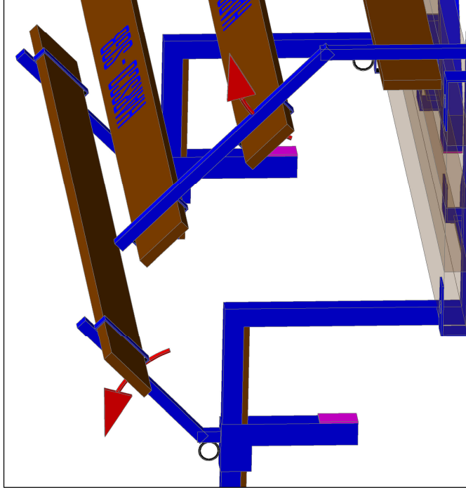
2. Dépliage des garde-corps
